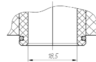
A-A увеличено
