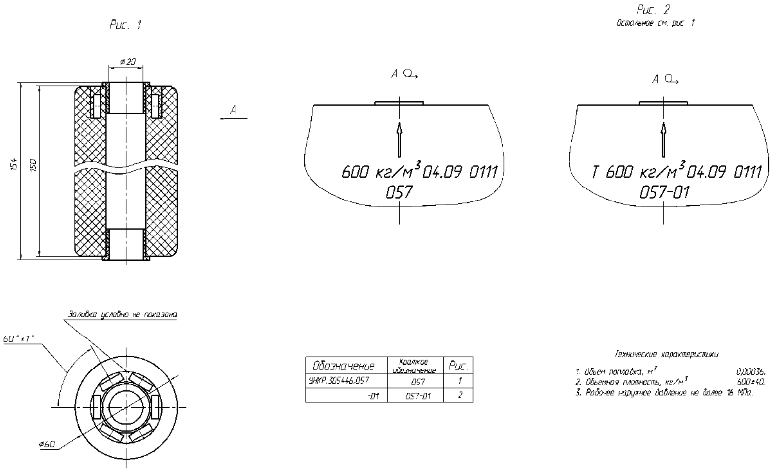
Рисунок А.9 - Габаритные размеры поплавка УНКР.305446.057
