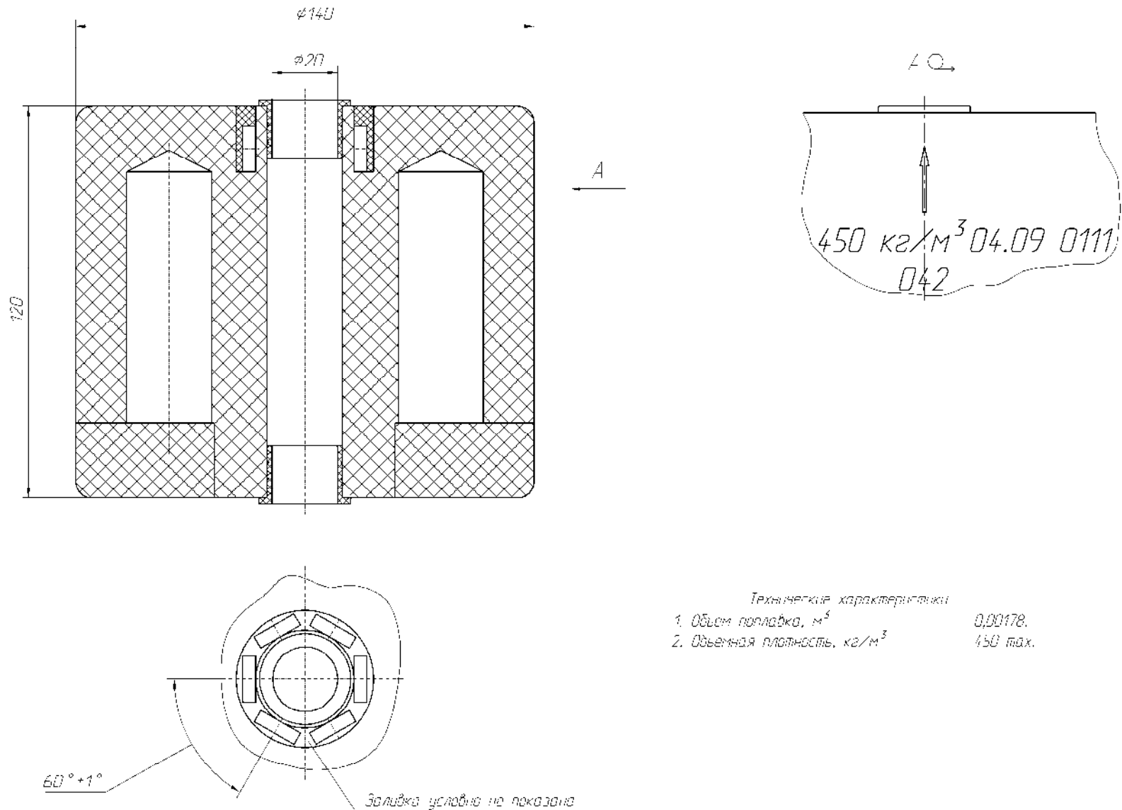
Рисунок А.7 - Габаритные размеры поплавка УНКР.305446.042
