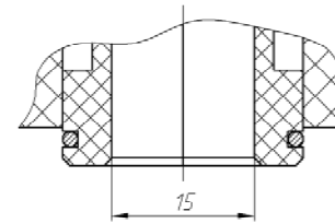
A-A увеличено
